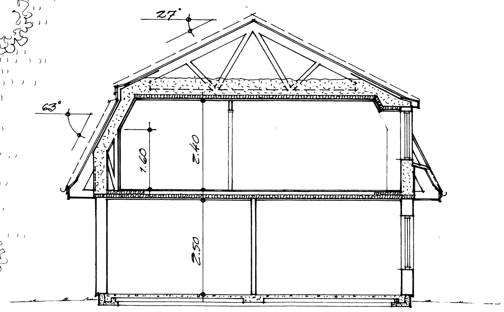
SEKTION
