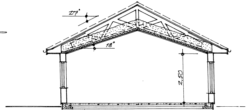
SEKTION, SNITT A
