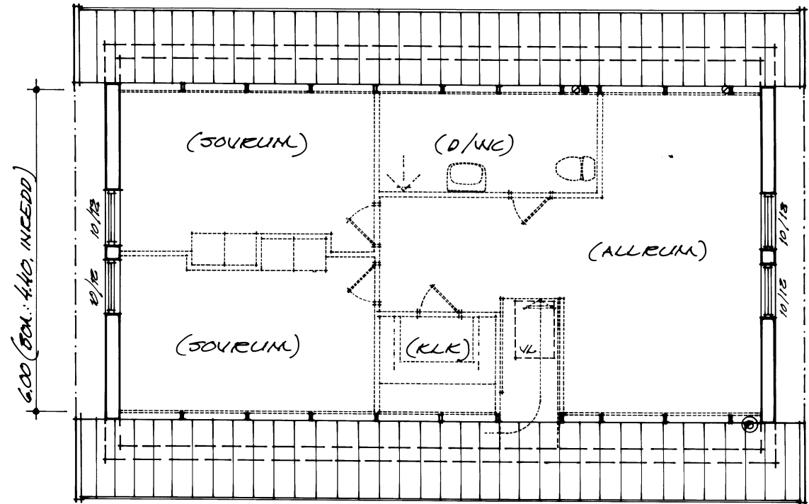
ÖVERPLAN, OINREDD, FÖRSLAG TILL DISPONERING BOAREÅ: 50.6 M 2 , INREDD. RÖRDRAGNING FÖRBEREDD.
