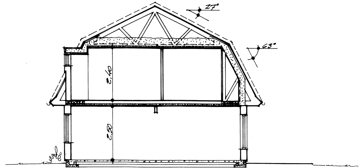
A-A SEKTION, SNITT A-A
