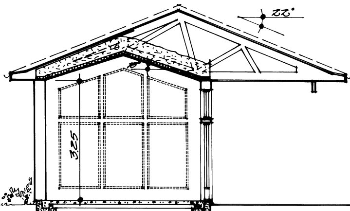
SEKTION VARDAGSRUM.
