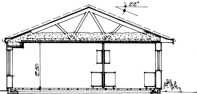
SEKTION MATPLATS/KÖK - KLÄVVARD.
