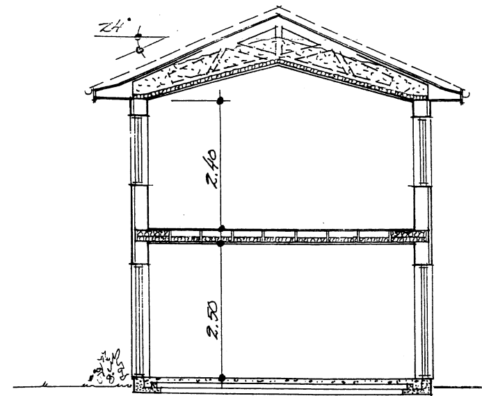
SEKTION, SNITT B-B
