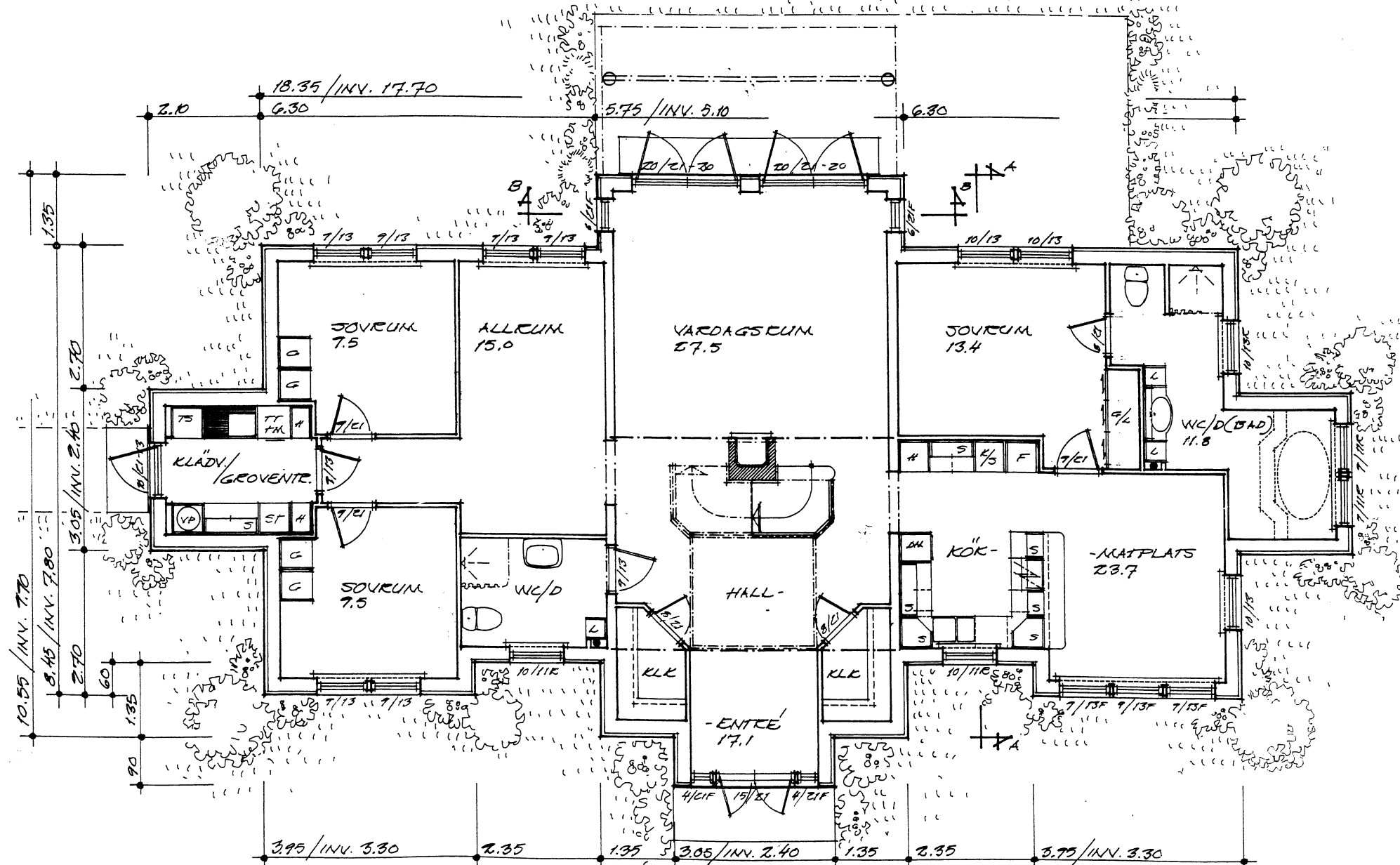
BOTTENPLAN BOAREA: 157.4 M 2 BYGGNADSYTA: 195.0 M 2
