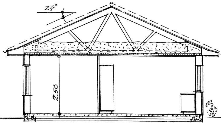
SEKTION, SNITT A-A.
