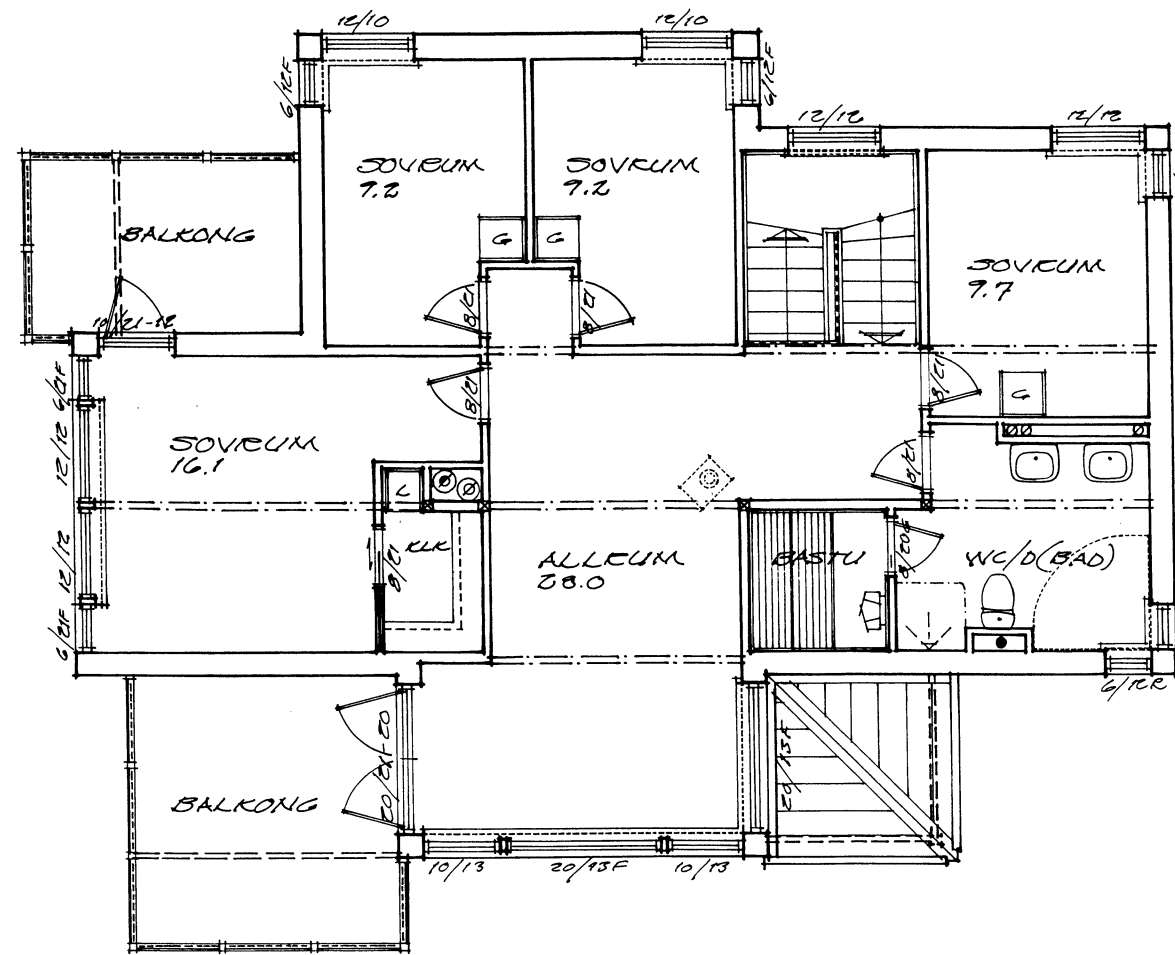
ÖVERPLAN BOAREAL: 73.6 M 2 .
