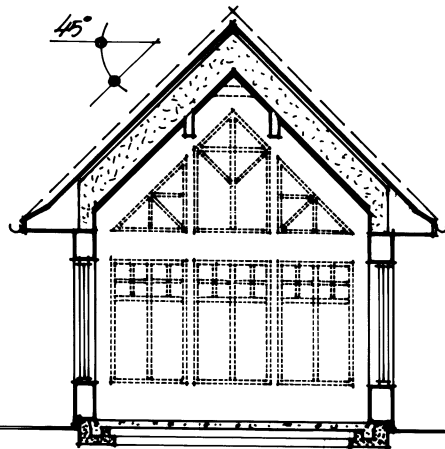
SEKTION VARDAGSRUM
